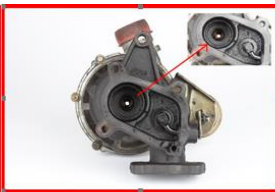
Figura 2 – Turbosuflyanta dezasamblata
